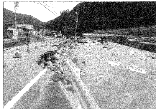
小野地区殿町の崩落した県道の護岸。県道と接続する崩落した露木橋。
